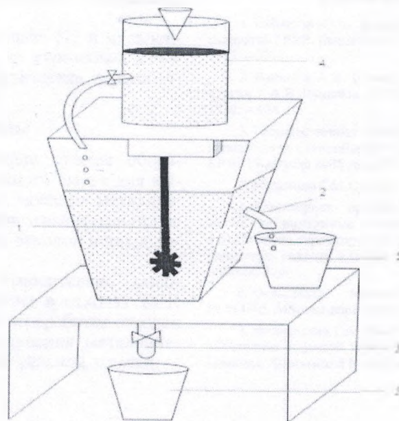
Гравитационный сепаратор: 1 – электромеханическая мешалка; 2 – сливной кран легкой фракции(классификатор); 3 – сливной кран тяжелой фракции; 4 – емкость для воды; 5 – емкость для отходов
