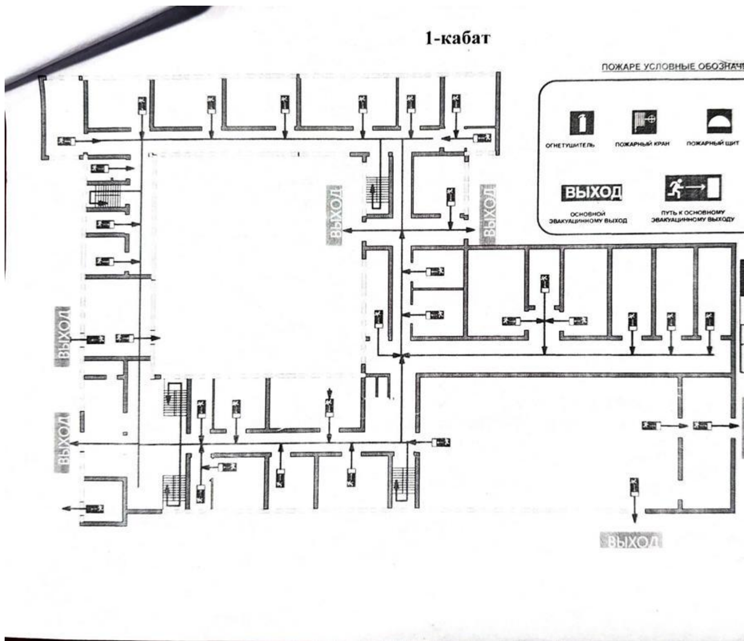
5.1. № 6.А Имараттын 1-кабатынын эскизи (каананын номерин, тепкич аянтчасын, коридорду, фойени, залды ж.б. көрсөтүү менен)
