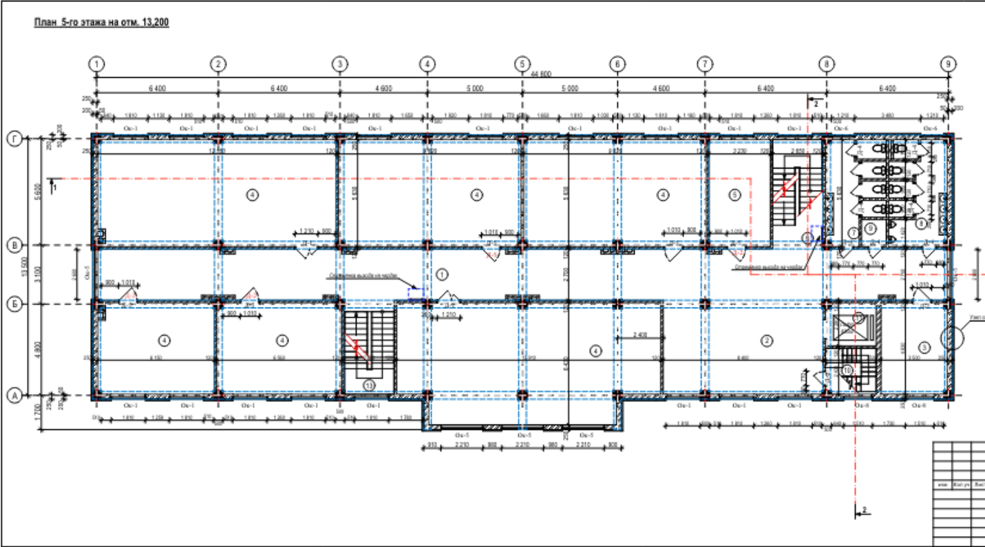
6.1. № 6.Б Имараттын 5-кабатынын эскизи (каананын номерин, тепкич аянтчасын, коридорду, фойени, залды ж.б. көрсөтүү менен)
